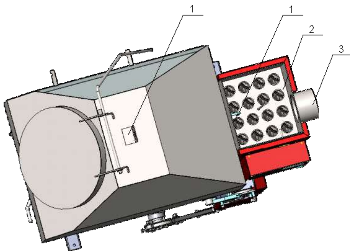
Рис.2. Вид теплообменника
