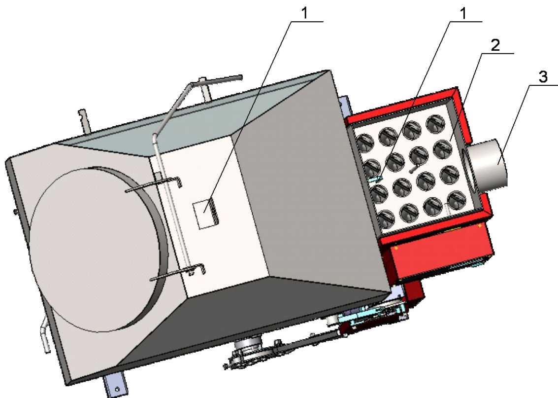
Рис.2. Вид теплообменника
