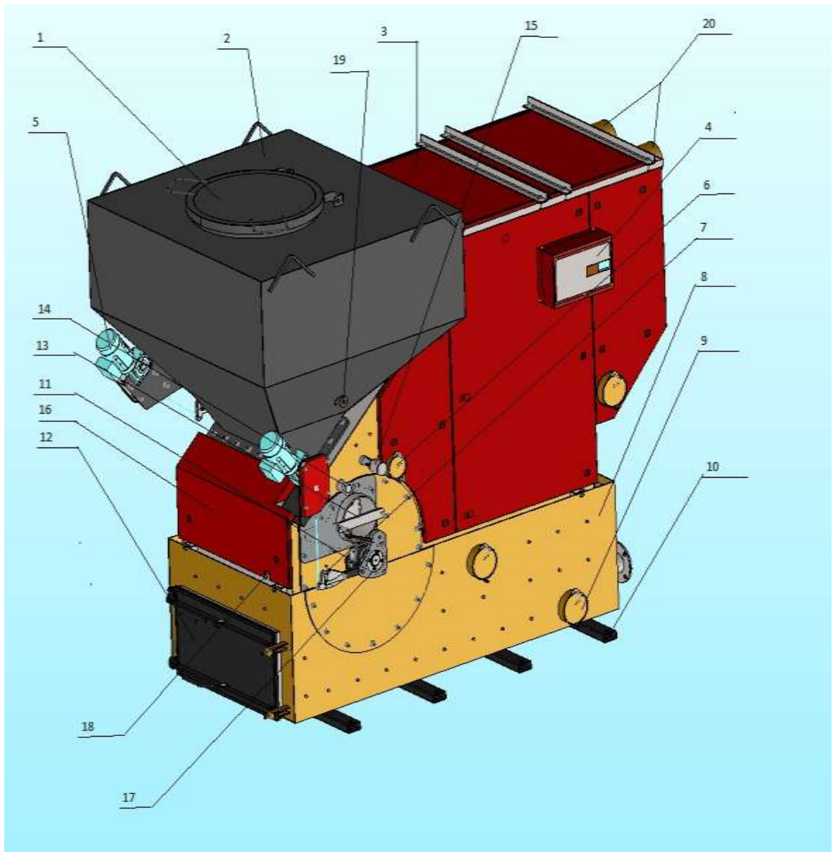
Рис.1. Внешний вид котла
