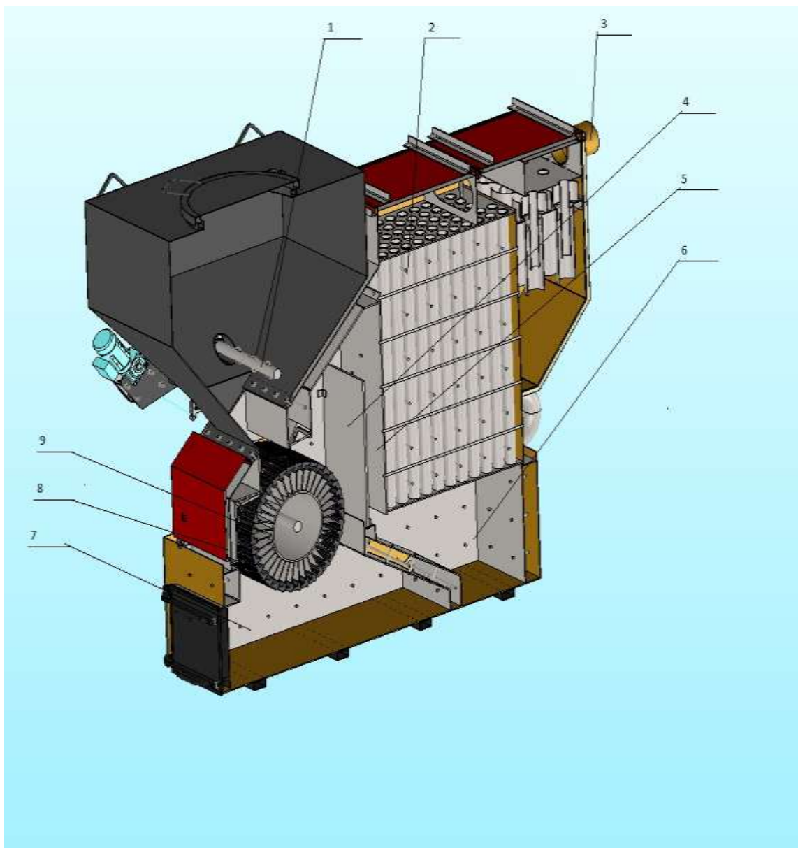
Рис.3. Котёл в разрезе
