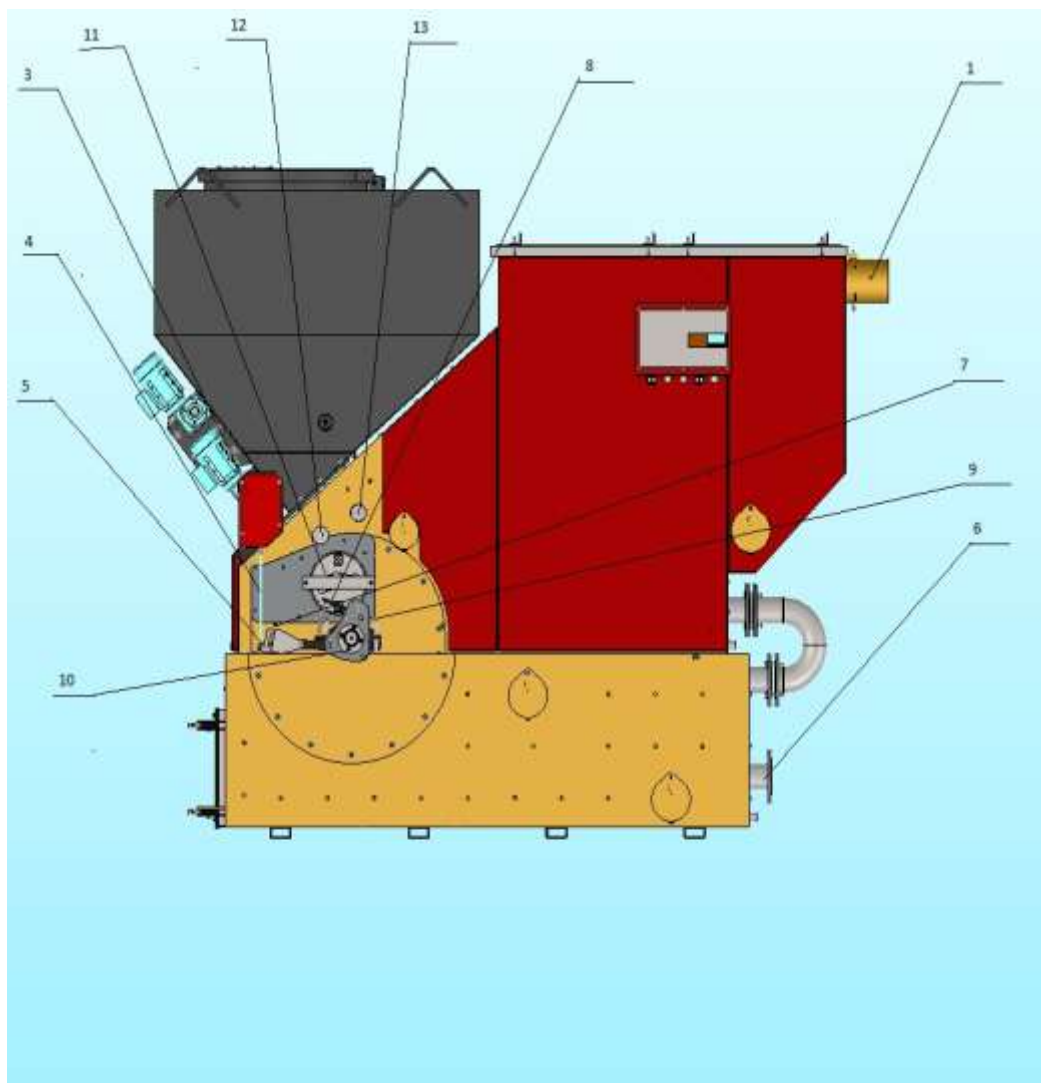
Рис.4. Расположение органов привода котла
