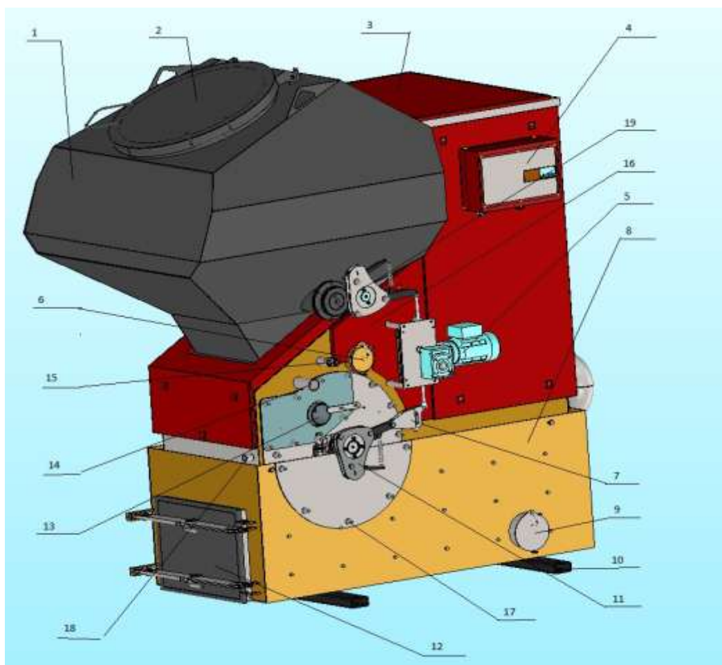
Рис.1. Внешний вид котла
