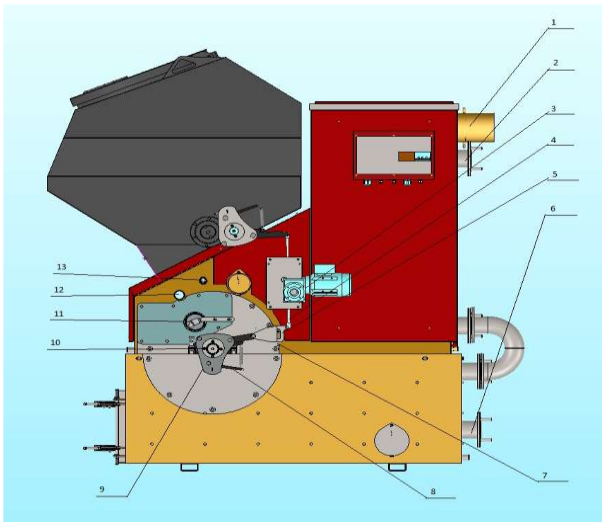
Рис.4. Расположение органов привода котла
