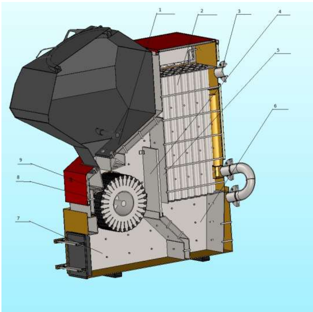
Рис.3. Котёл в разрезе
